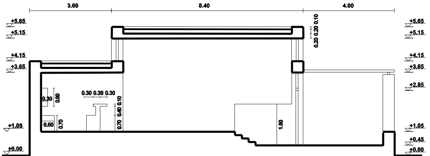
ΤΟΜΗ Α-Α
