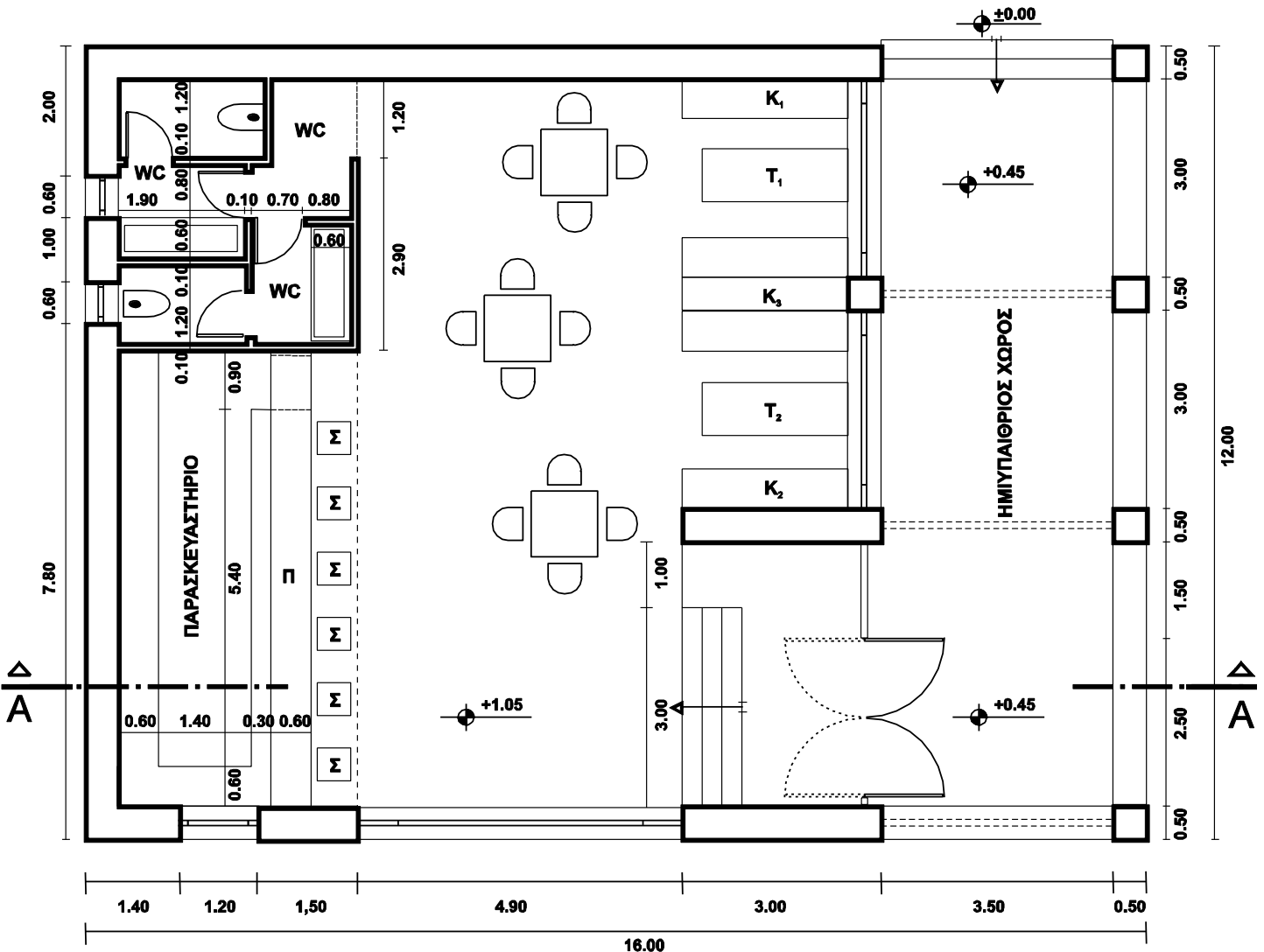
ΚΑΤΟΨΗ
